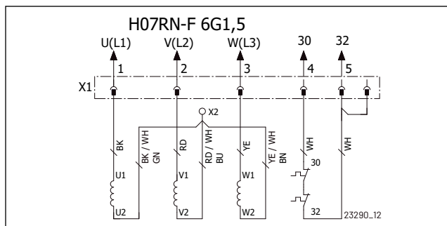
Y-Circuito, alta tensione
