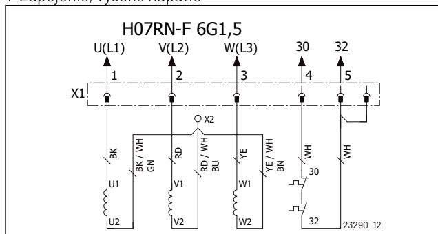
Y-Zapojenie, vysoké napätie
