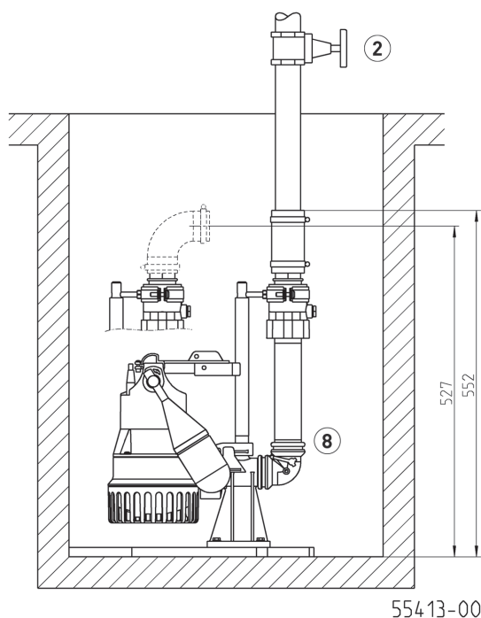
Einbaubeispiel und Hauptmaße Easyfix 32 Single
